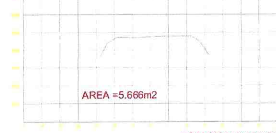
ESTACION 0+550.00
