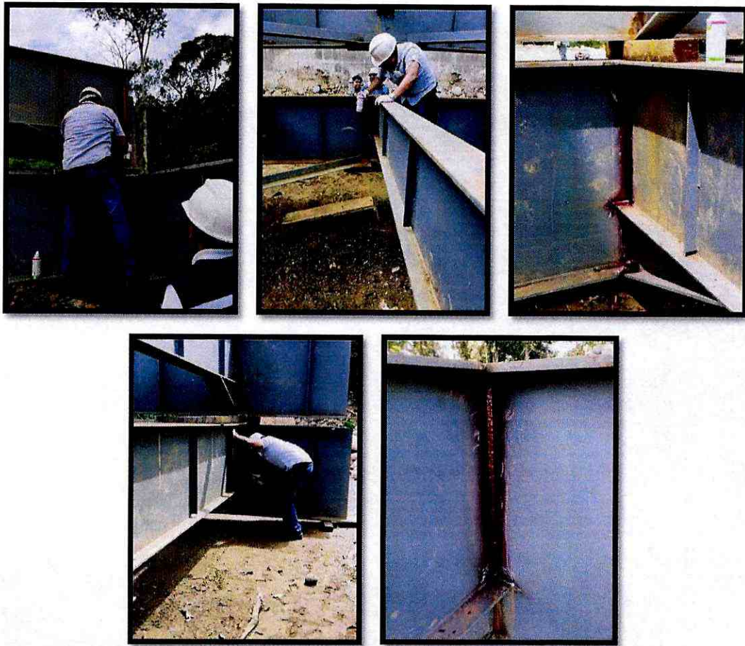
6.- Aplicación de la tinta penetrante
