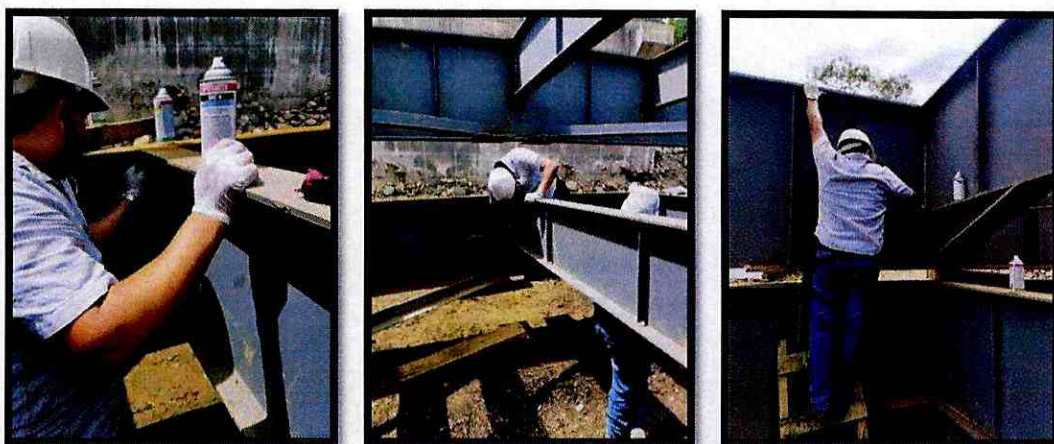
7.- Limpieza del exceso de tinta penetrante.
