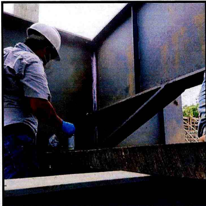
Fotografía 4. Ensayo de tintas penetrantes
