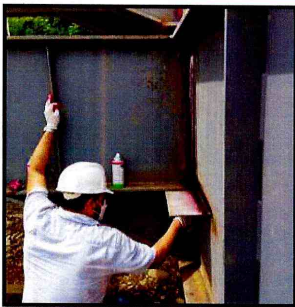
Fotografía 5. Ensayo de tintas penetrantes
