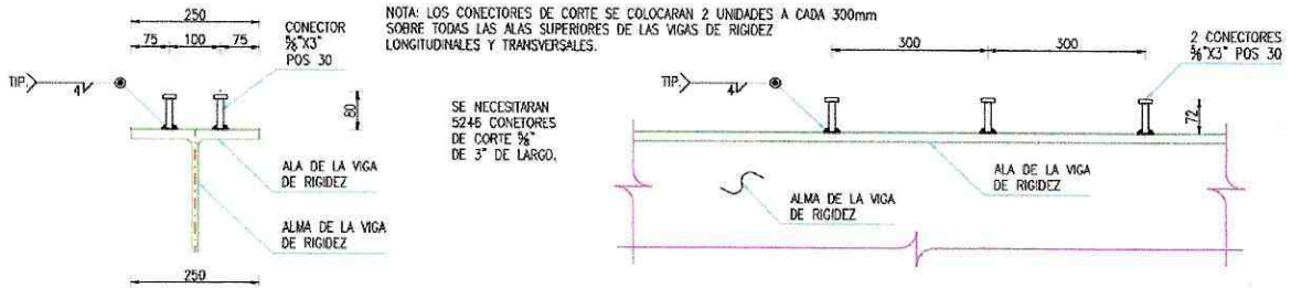
DETALLE DE GEOMETRIA Y SOLDADURA DE CONECTORES DE CORTE ESCALA 1:10
