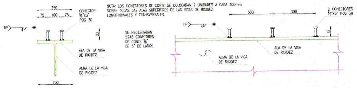
DETALLE DE GEOMETRIA Y SOLDADURA DE CONECTORES DE CORTE ESCALA 1:10
