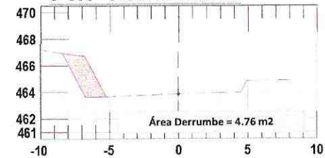
3+500 - 3+560 / Derrumbe
