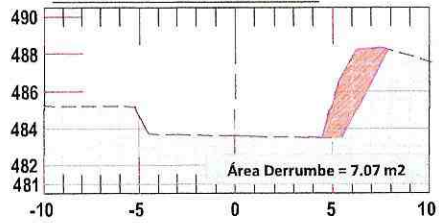
1+100 - 1+140 / Derrumbe
