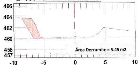
3+500 - 3+560 / Derrumbe
