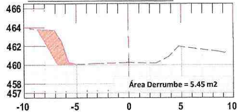
3+500 - 3+560 / Derrumbe
