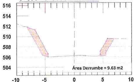
2+090 - 2+130 / Derrumbe
