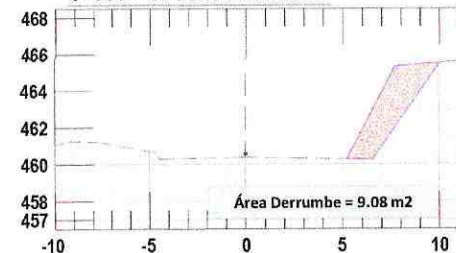
4+005 - 4+143 / Derrumbe
