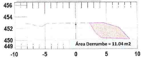
3+050 - 3+070 / Derrumbe
