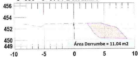
3+050 - 3+070 / Derrumbe
