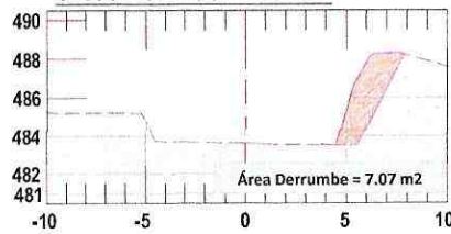
1+100 - 1+140 / Derrumbe
