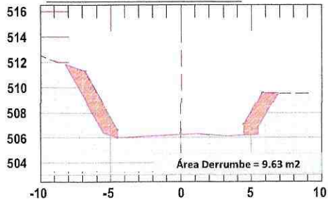
2+090 - 2+130 / Derrumbe
