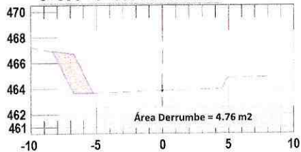
3+500 - 3+560 / Derrumbe
