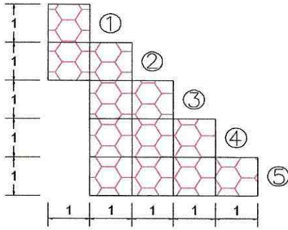
MURO DE GAVIONES ABCISIA 3+060
