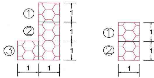
MURO DE GAVIONES ABCISIA 4+400
