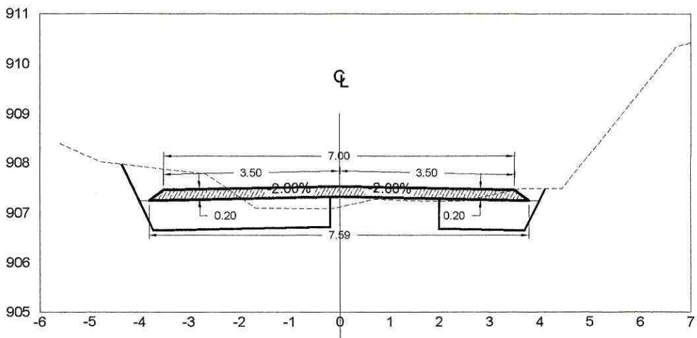
ESTACION 2+160.00 ESCALA HORIZONTAL 1 : 100 ESCALA VERTICAL 1 : 100
