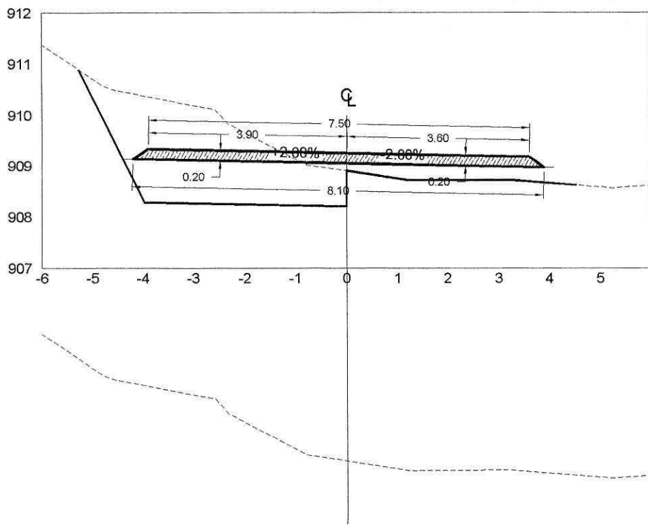
ESTACION 2+200.00 ESCALA HORIZONTAL 1 : 100 ESCALA VERTICAL 1 : 100
