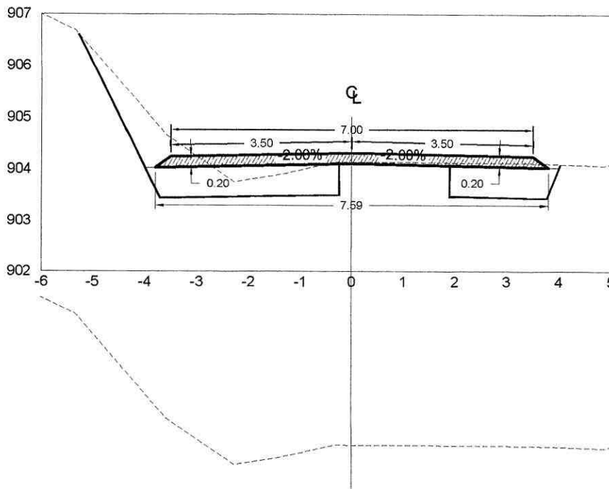
ESTACION 2+100.00 ESCALA HORIZONTAL 1 : 100 ESCALA VERTICAL 1 : 100
