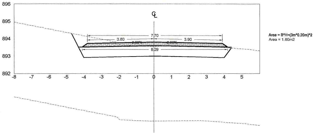
ESTACION 1+940.00 ESCALA HORIZONTAL 1 : 100 ESCALA VERTICAL 1 : 100
