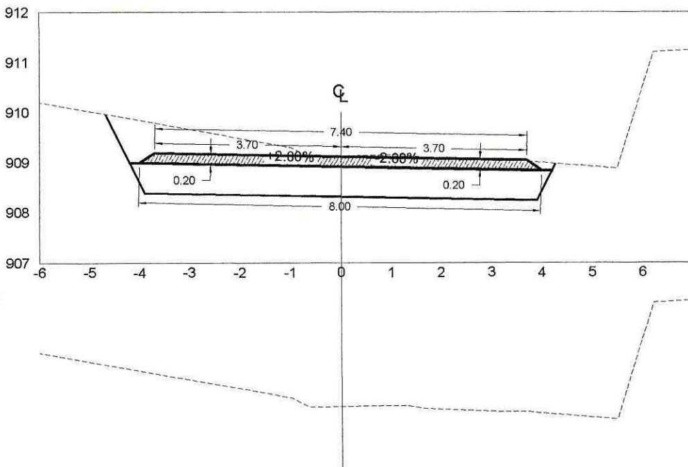
ESTACION 2+200.00 ESCALA HORIZONTAL 1 : 100 ESCALA VERTICAL 1 : 100
