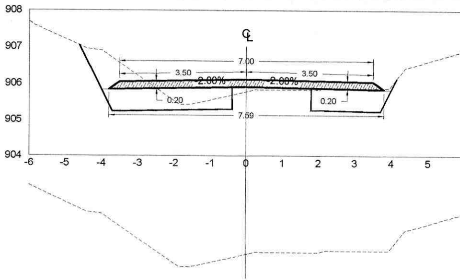
ESTACION 2+120.00 ESCALA HORIZONTAL 1 : 100 ESCALA VERTICAL 1 : 100
