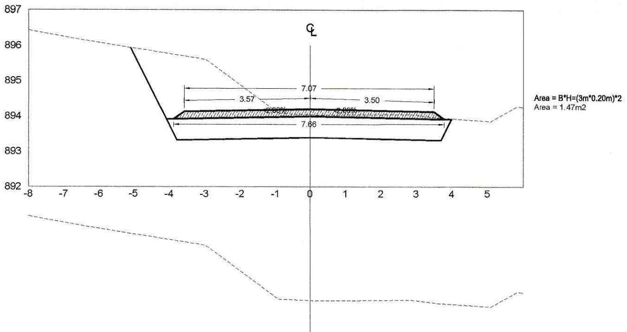
ESTACION 1+940.00 ESCALA HORIZONTAL 1 : 100 ESCALA VERTICAL 1 : 100
