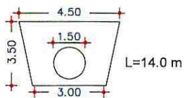
Excavación y Relleno en Abscisa 3+400 en Tubería Metálica D=1.50m
