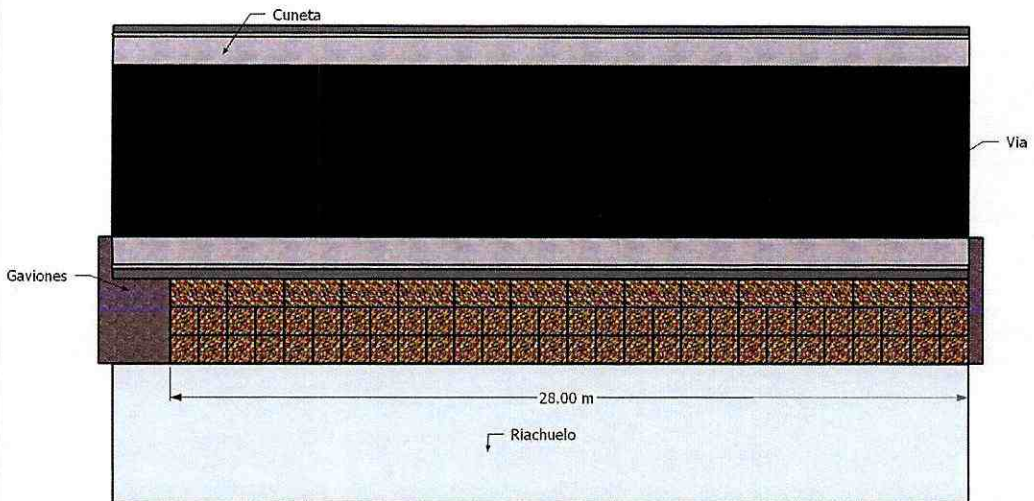
Muro de Gaviones desde abscisa 2+412 hasta 2+440
