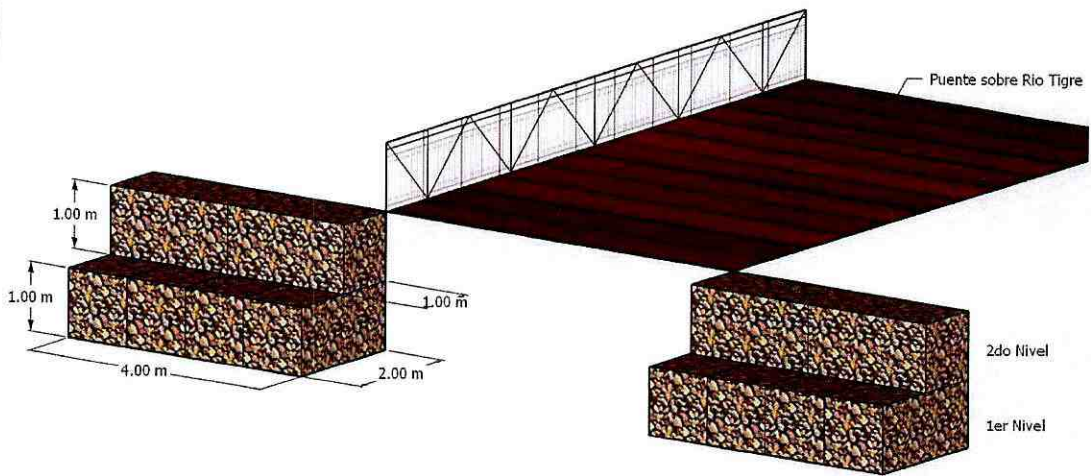
Muro de Gaviones en abscisa 0+570
