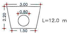
Excavación y Relleno en Abscisa 3+115 en Tubería Metálica D=0.80m
