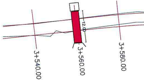
Alcantarillas en abscisas 3+560
