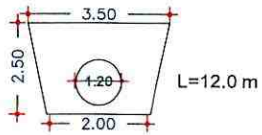
Excavación y Relleno en Abscisa 3+070 en Tubería Metálica D=1.2m
