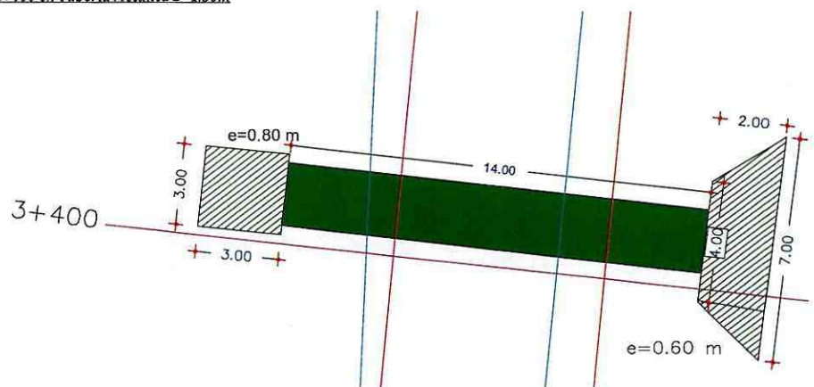
Excavación y Relleno en Abscisa 3+400 en Tubería Metálica D=1.50m
