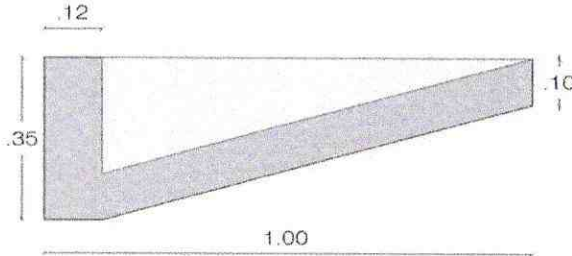
EXCAVACIÓN PARA CUNETA (A = 0.24 m 2 )
