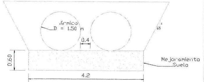
Sección Exc. y Pelleno (Tub. D=1.50 m)
