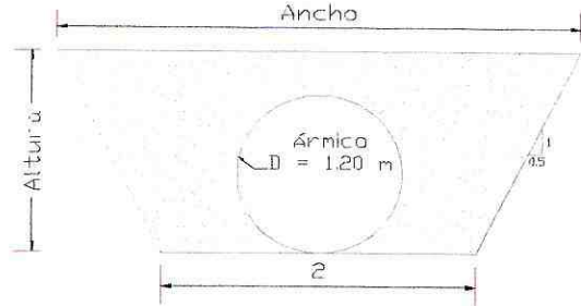
Sección Relleno (Tub. D=1.20 m)
