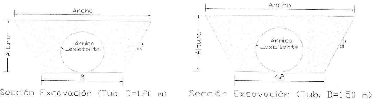
GRÁFICO Sección de excavación para colocación de ármicos
