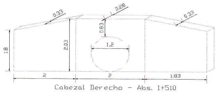
Dimensiones de cabezales derrocados ABS 1+510
