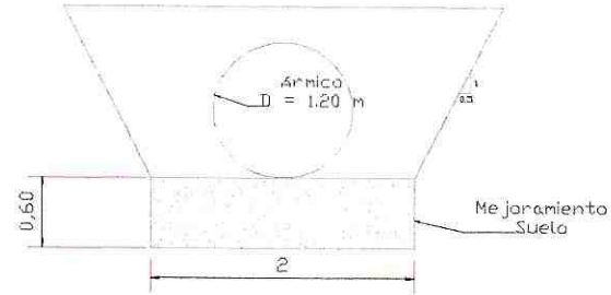
Sección Exc. y Pelleno (Tub. D=1.20 m)
