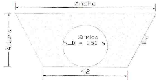
Sección Relleno (Tub. D=1.50 m)
