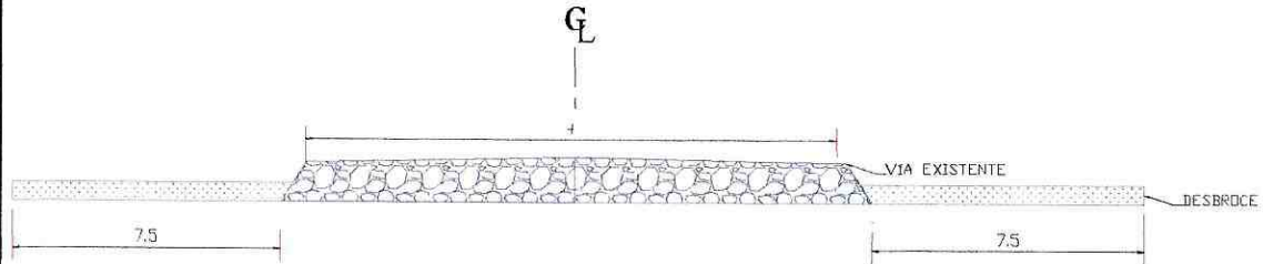
GRÁFICO Sección de desbroce, desbosque y limpieza
