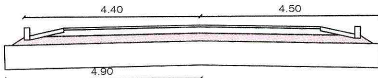
SECCIÓN TIPO 3: Área=1.70
