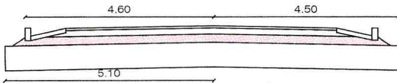
SECCIÓN TIPO 6: Área=1.74
