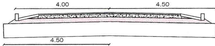
SECCIÓN TIPO 9: Área=1.62
