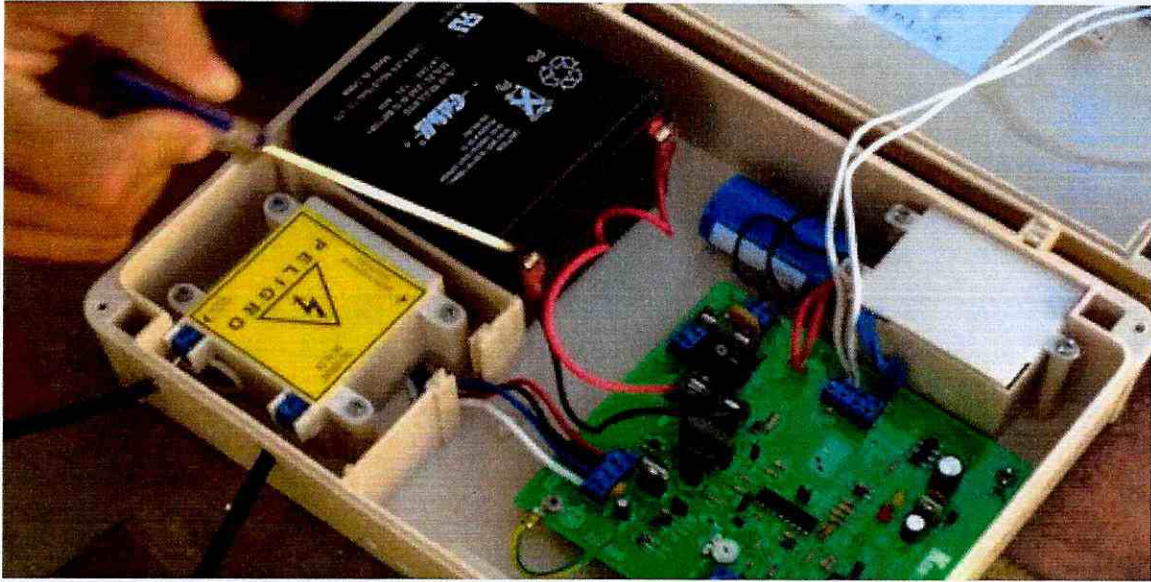
INSTALACION DE CENTRAL ENERGIZADORA 5K
