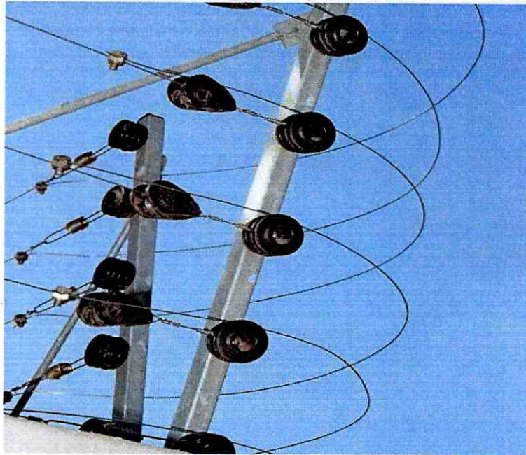
COLOCACION DE AISLADORES DE PASO DE ESQUINA Y PASANTE
