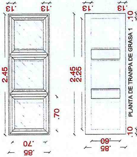
PLANTA DE TRANPA DE GRASA 1 MEC. LIVIANA
