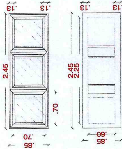
PLANTA DE TRANPA DE GRASA 1
