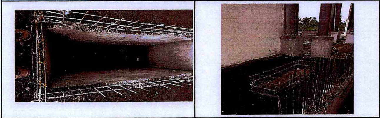
HORmIGON PREmEZCLADO COLUmNAS F'C=280 KG/Cm2 INC. ENCOFRADO, BOMBA Y TRANSPORTE
