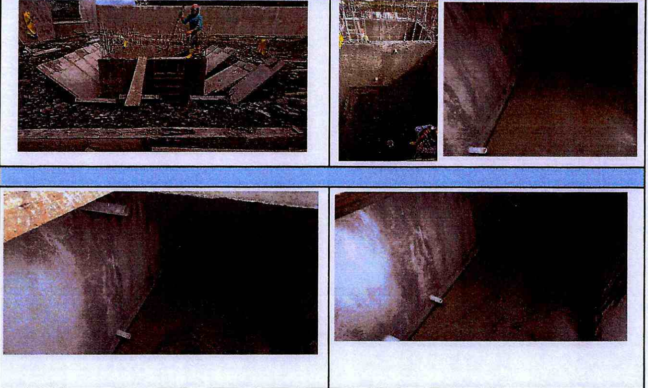
ENLUCCIDO CON IMPERMEABILIZANTE MORTERO 1:3 (EXTERIOR)
