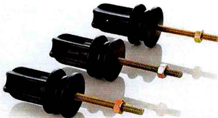
COLOCACION DE AISLADORES DE PASO DE ESQUINA Y PASANTE
