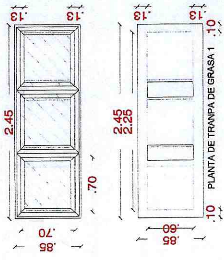
PLANTA DE TRANPA DE GRASA 1 MEC. LIVIANA
