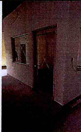
Puerta batiente aluminio y vidrio flotado claro 6mm (1.00x2.10)
