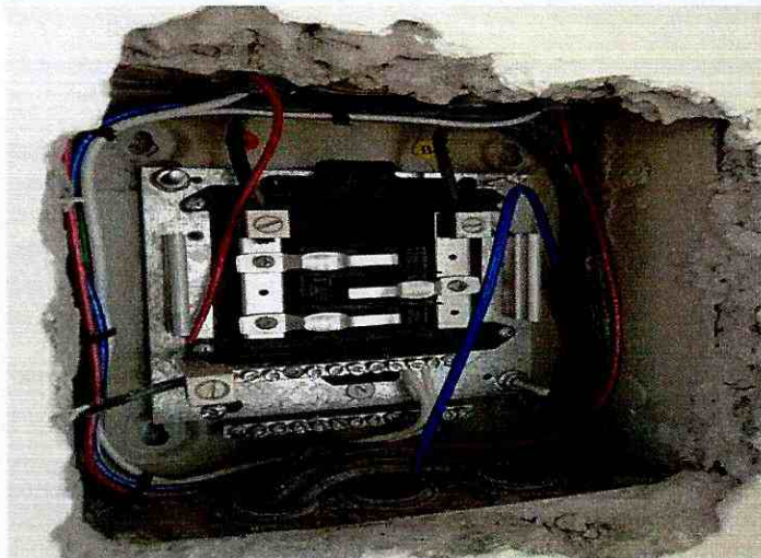
TENDIDO DE CABLE FLEXIBLE DE COBRE NO.10 AWG COLOR AZUL (INC. TAYPE)
