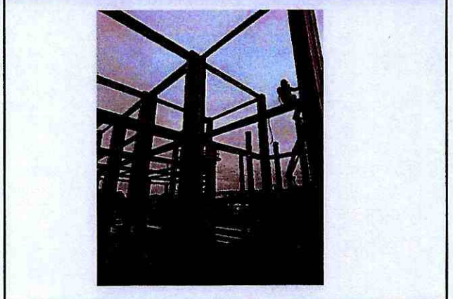
TRATAMIENTO PINTURA ESTRUCTURA ACERO A36 (FONDO+PINTURA ANTICORROSIVA), A COMPRESOR
