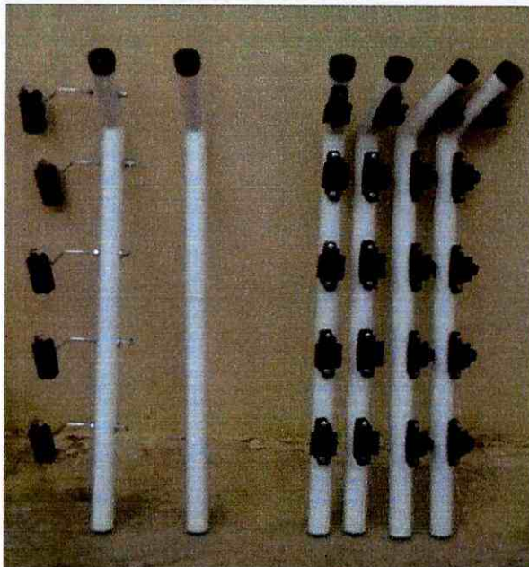
COLOCACION DE TuBERIA PREPARADA
