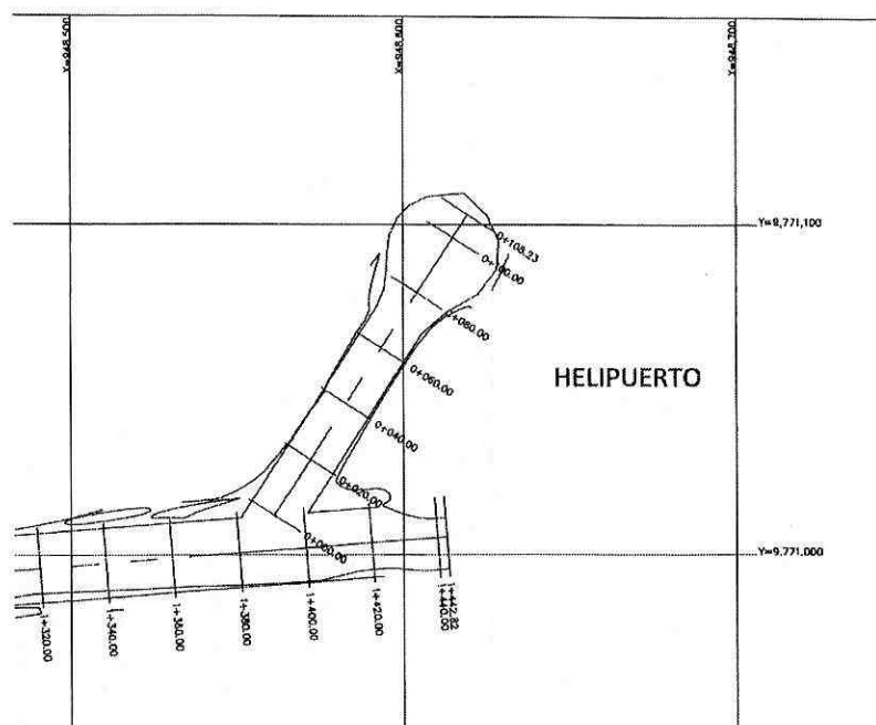
Ilustración 2. Plano topográfico PRELIMINAR. Levantamiento del lugar.
