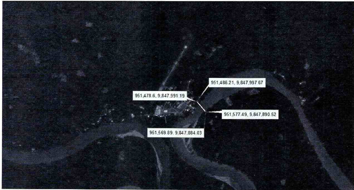
Ilustración 2, Ubicación del puente usando coordenadas UTM WGS84- Z 17S, Arcgis
